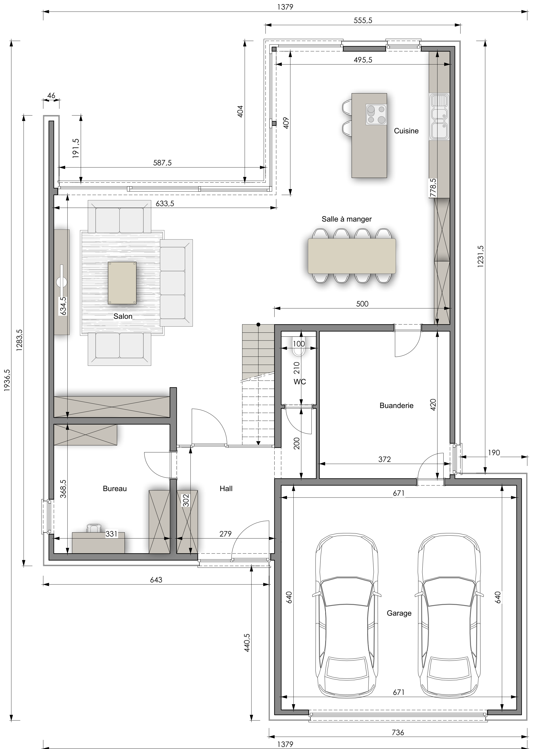
PLAN REZ-DE-CHAUSSEE
