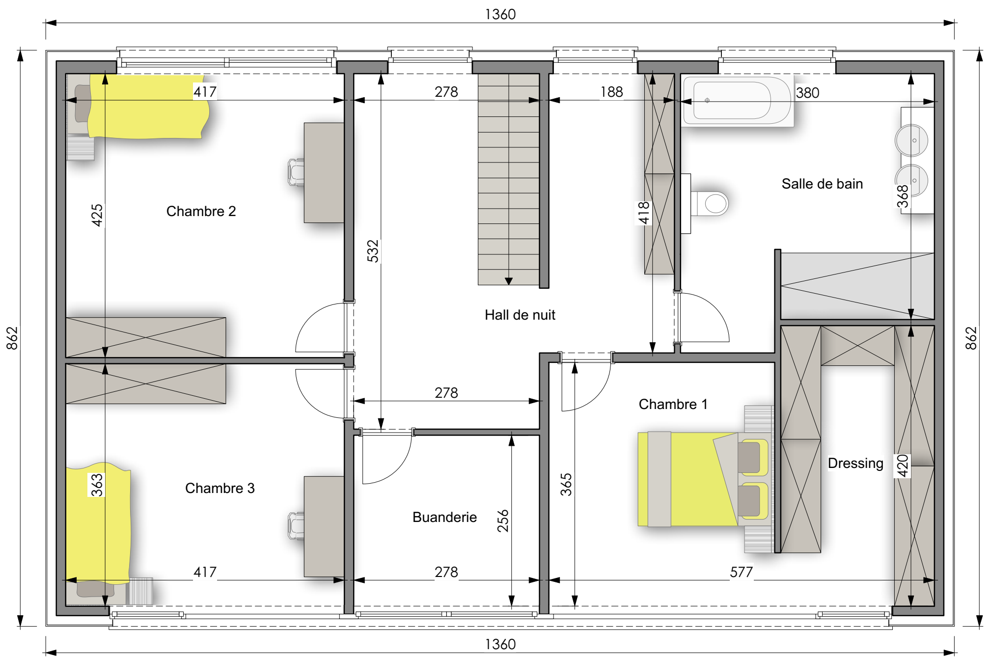
PLAN PREMIER ETAGE
