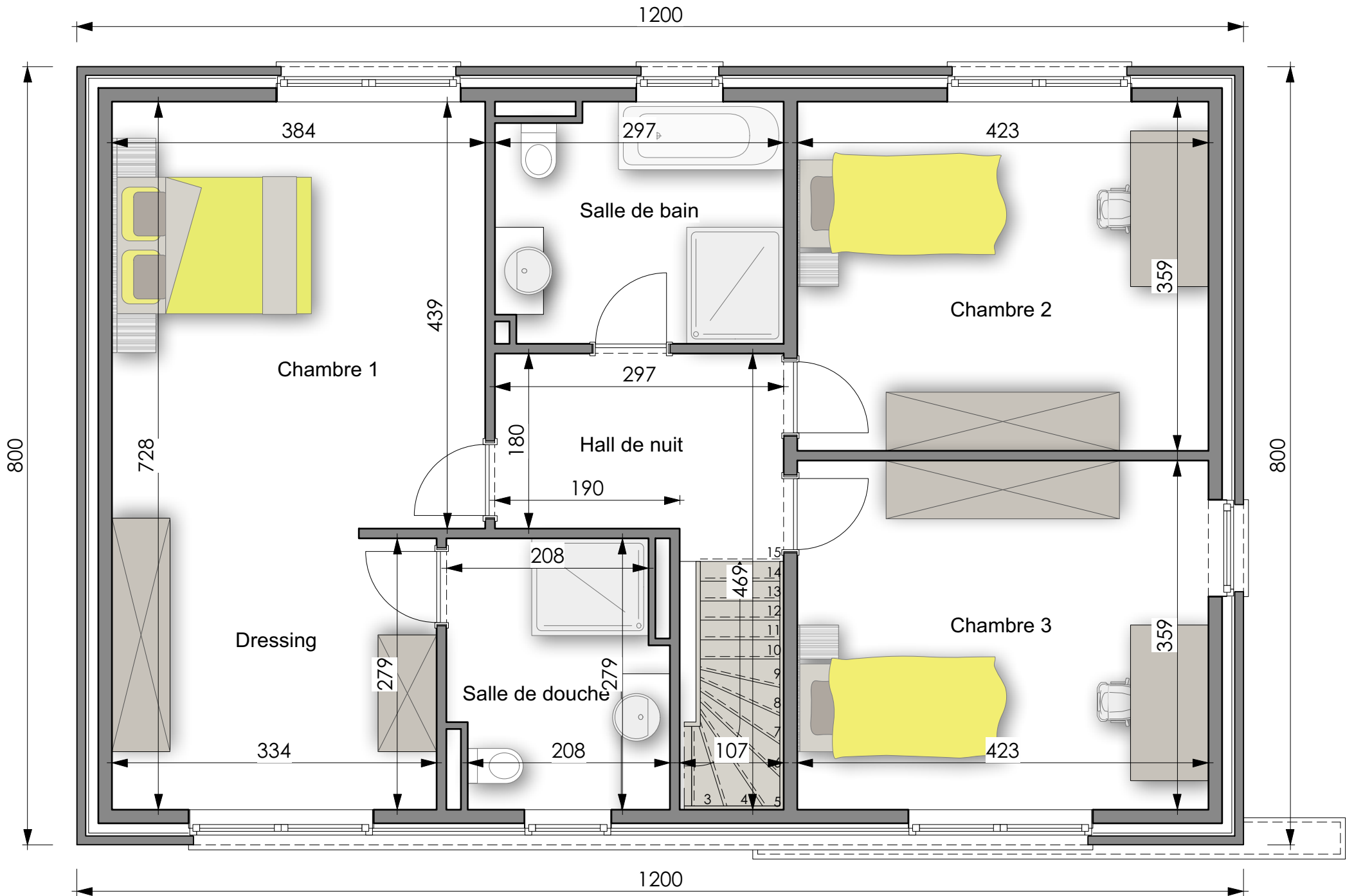
PLAN PREMIER ETAGE
