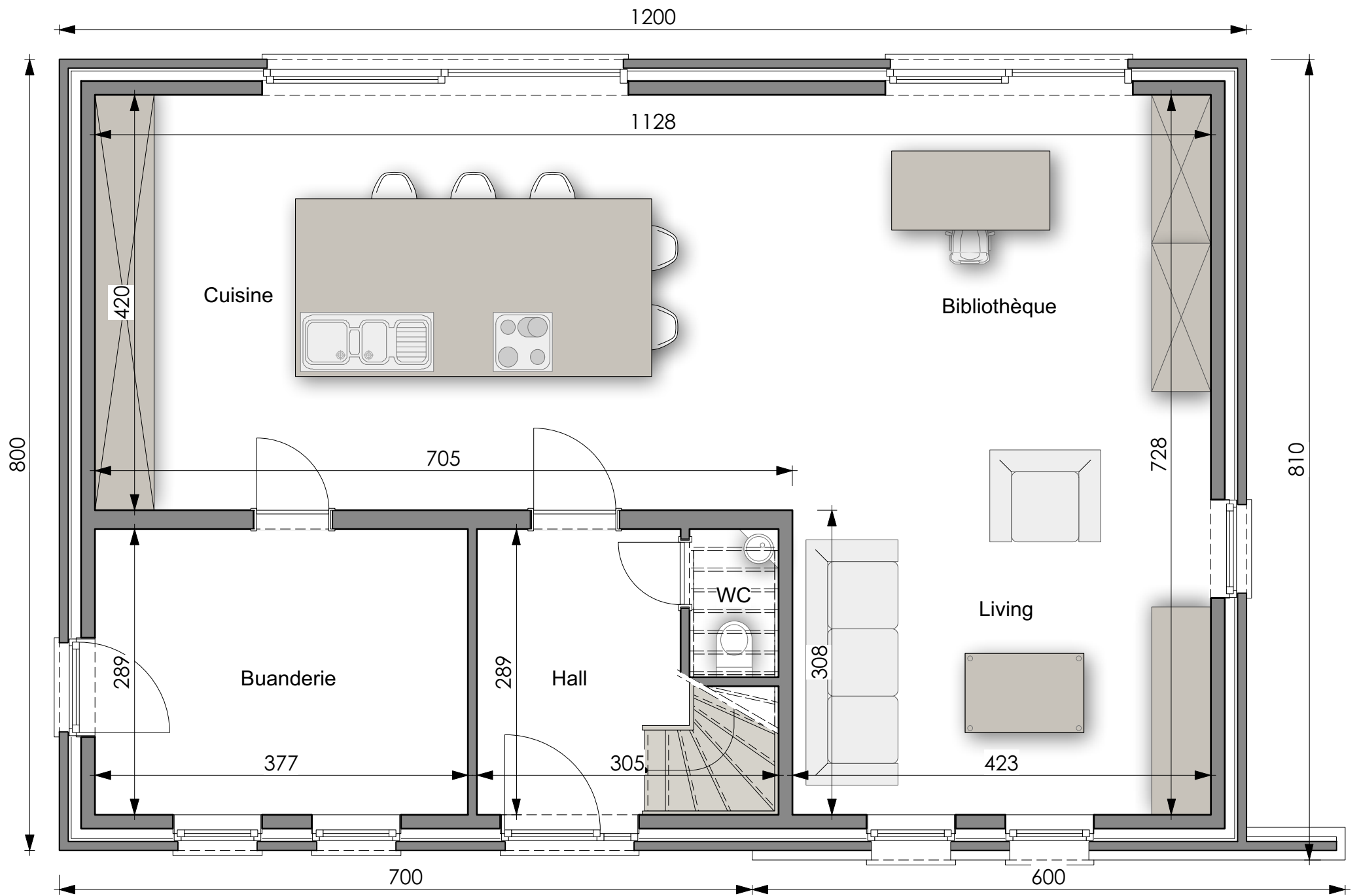
PLAN REZ-DE-CHAUSSEE
